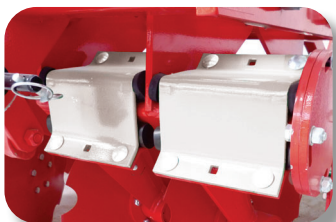
Système Non Stop à base d'élastomères avec reliefs anti-expulsion.
