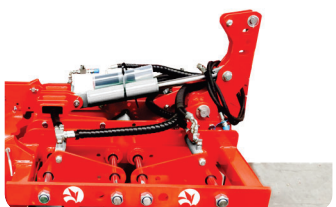
Châssis relevable hydrauliquement pour une meilleure maniabilité en bout de champ.
