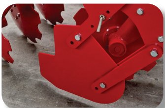
Plaques limitatrices latérales avec parallélogramme.
