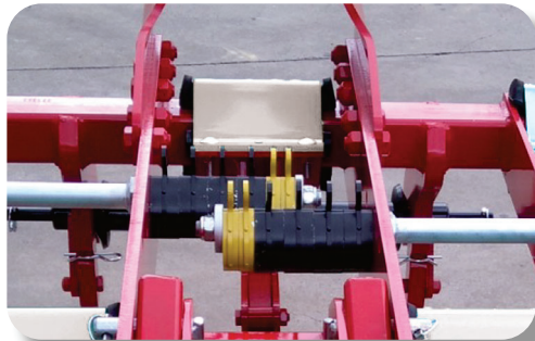
Châssis télescopique manuel au lieu d'hydraulique. Grande facilité et confort grâce au système de clips.
