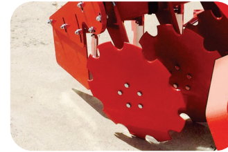
Disques de 20" (510 mm) en 6 mm d'épaisseur.
